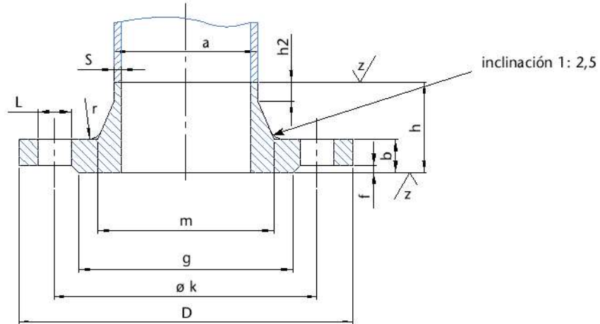
DIN 2634 PN25 ; DIN 2635 PN40
